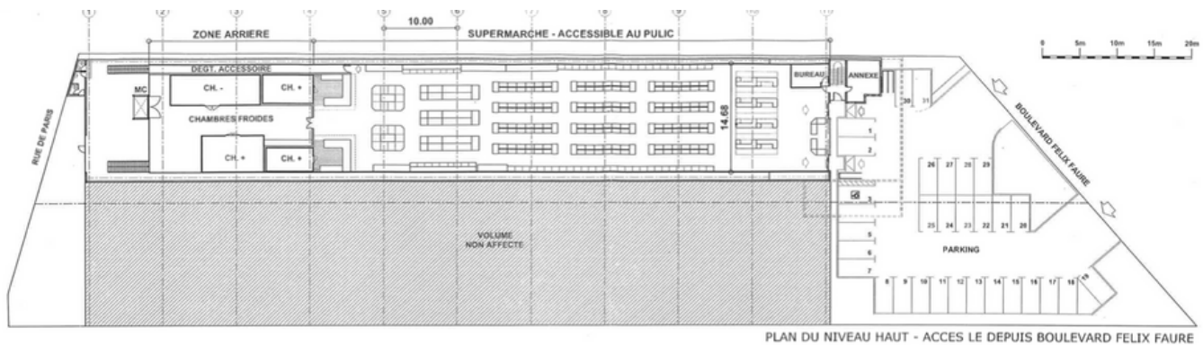
PLAN DU NIVEAU HAUT - ACCES LE DEPUIS BOULEVARD FELIX FAURE
